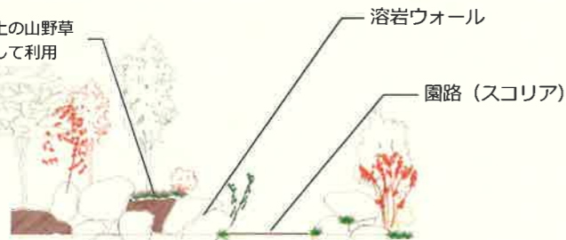
A-A 断面
